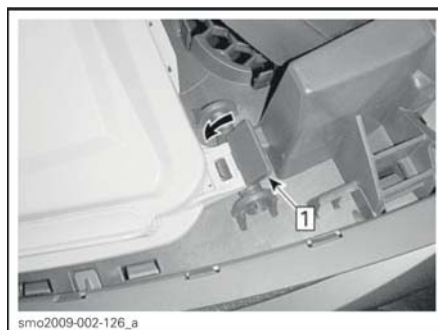
Шаг 1: Нажмите на защелки для закрепления
