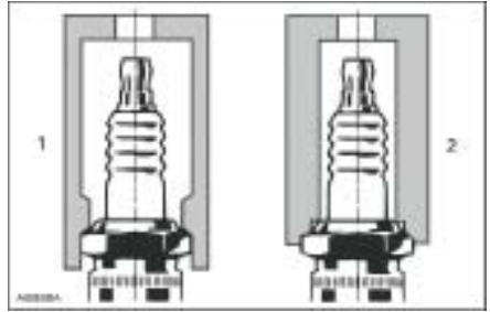
1. Разрешенный к использованию ключ
