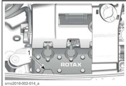
ТИПОВОЙ ВАРИАНТ – ДЛЯ ДВИГАТЕЛЕЙ 300
