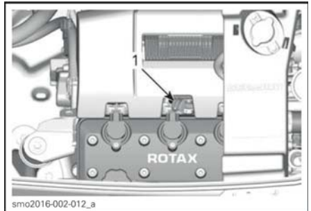
ТИПОВОЙ ВАРИАНТ – ДЛЯ ДВИГАТЕЛЕЙ 300
