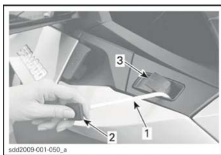
ТИПОВОЙ ВАРИАНТ - НОСОВОЙ ШВАРТОВ
