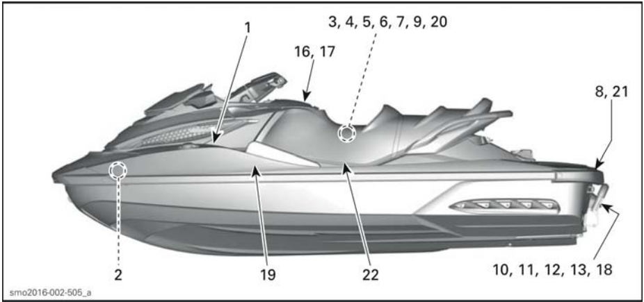
ТИПОВОЙ ВАРИАНТ – МОДЕЛИ GTx LIMITED 300
