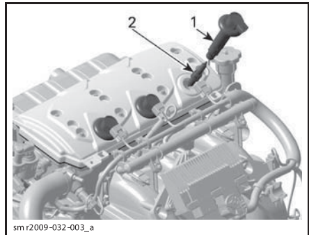
1. Катушка зажигания
