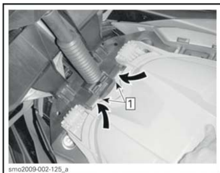
Шаг 1: Установите выступы контейнера
