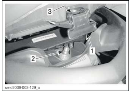
ТИПОВОЙ ВАРИАНТ – ЗАЩЕЛКА СИДЕНЬЯ
