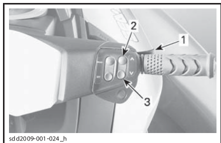
ТИПОВОЙ ВАРИАНТ – ИЗМЕНЕНИЕ ЗАДАННОЙ СКОРОСТИ КРУИЗ-КОНТРОЛЯ
