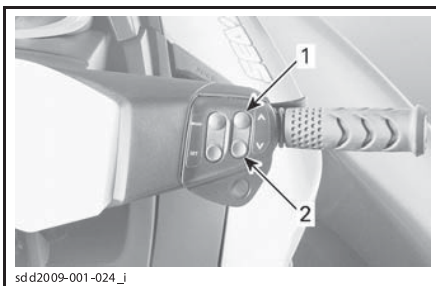
ТИПОВОЙ ВАРИАНТ – РЕГУЛИРОВКА НЕЙТРАЛЬНОГО ПОЛОЖЕНИЯ ОТРАЖАТЕЛЯ СИСТЕМЫ iBR
