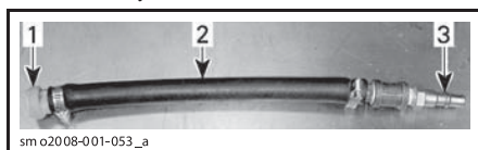
ТИПОВОЙ ВАРИАНТ 1. Переходник для промывочного штуцера 2. Шланг 12,7 мм 3. Переходник для источника сжатого воздуха
